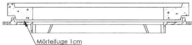
Darstellung mit Auflagering nach DIN V 4034-1
